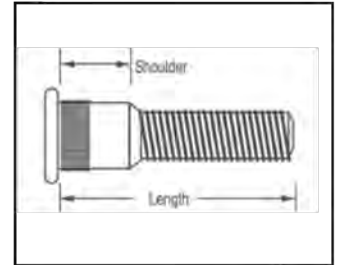
HUB STUDS
